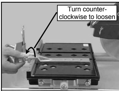
(D) Loosen the Adjustable Cutting Guide retaining thumbscrew
